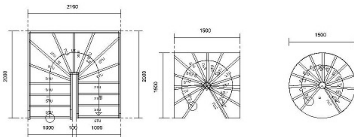
Treppe 3. 1 / 2 gewunden
